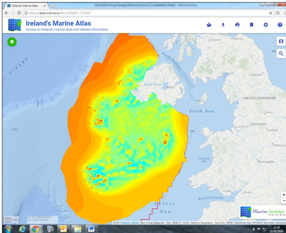
Figiúr 4: Luas na Gaoithe ag 100m Foinse: Sonraí ón téama acmhainní fuinnimh gaoithe ar féidir rochtain a fháil orthu trí Atlas Mara na hÉireann ag http://atlas.marine.ie/ [11/7/19]
